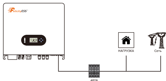
Рисунок 4.3-2 Подключение выключателя переменного тока
