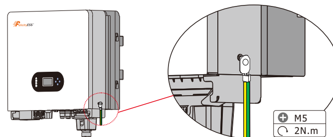
Рисунок 3.4- 3 Заземление стойки (заземляющий провод зафиксирован винтом M5)
