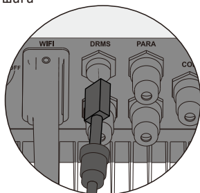
Рисунок 4.5-2 Этапы подключения
