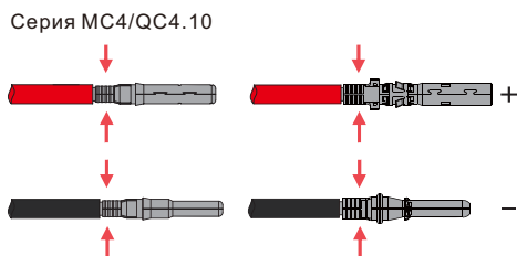
Рисунок 4.1-2 Соединение ФЭ кабелей с ФЭ разъемами
