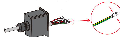
Рисунок 4.5-3 Установка соединительных клемм переменного тока
