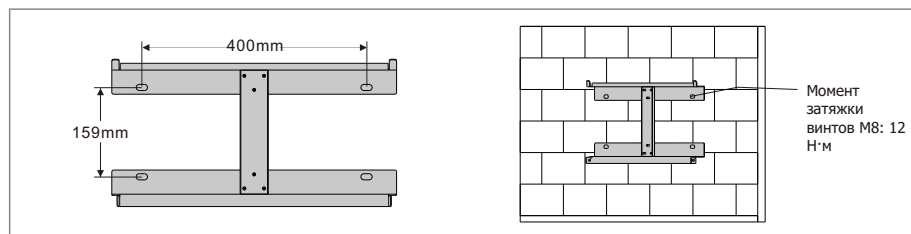
Рисунок 3.4-1. Установка настенной пластины инвертора
