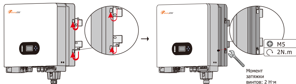
Рисунок 3.4-2. Установка инвертора
