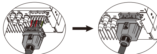
Рисунок 4.6-3 Установка соединительных клемм переменного тока
