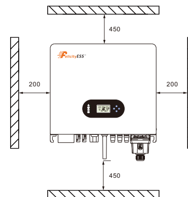
Рисунок 3.3-1 Пространство для установки одного инвертора
