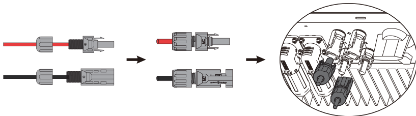
Рисунок 4.1-3. Подключение ФЭ-штекеров к разъемам инвертора
