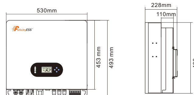
Рисунок 2.1-2 Габаритные размеры инвертора
