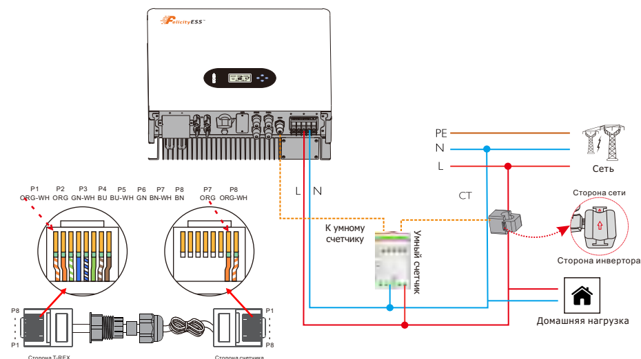
Рисунок 4.4-4 Подключение умного счетчика
