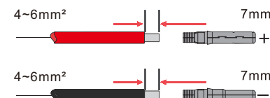
Рисунок 4.1-1 Кабели и штекеры ФЭ системы
