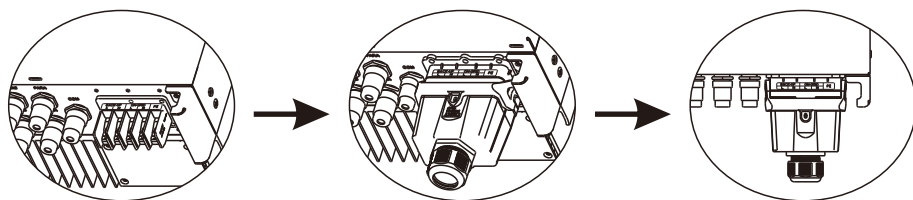
Рисунок 4.3-1 Установка кабелей переменного тока для инвертора
