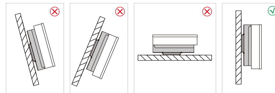
Рисунок 3.3-2 Положение при установке
