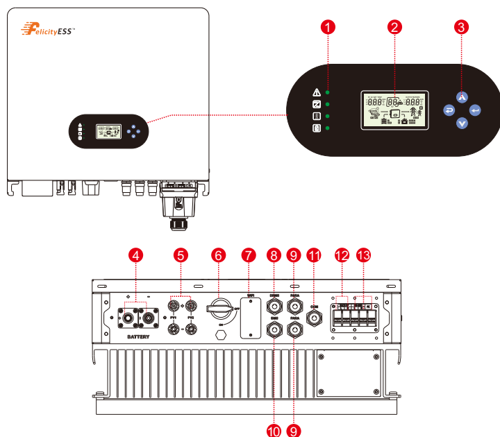
Рисунок 2.1-1 Обзор компонентов изделия
