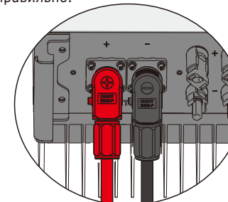
Рисунок 4.2-3 Подключение клемм аккумулятора к инвертору
