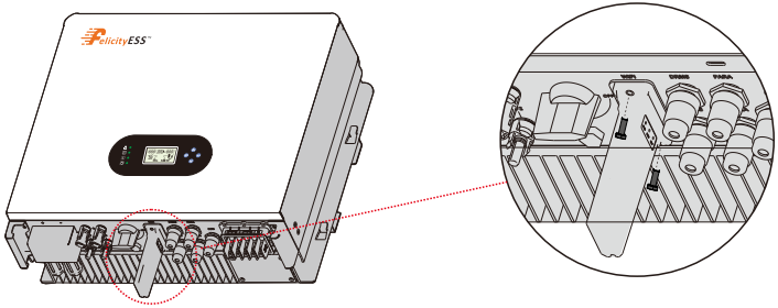
Рисунок 4.7-1 Установка модуля Wi-Fi
