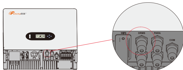
Рисунок 4.5-1 Интерфейс DRMS
