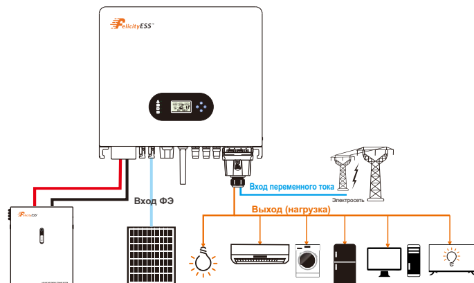
Рисунок 2. Функциональная схема гибридной солнечной инверторной системы
